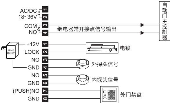
外接DC12V稳压电源接法示意图
