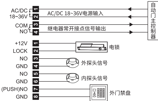
从自动门机组取AC/DC24V电源接法示意图
