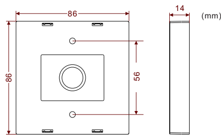
M-605M(明装款)
