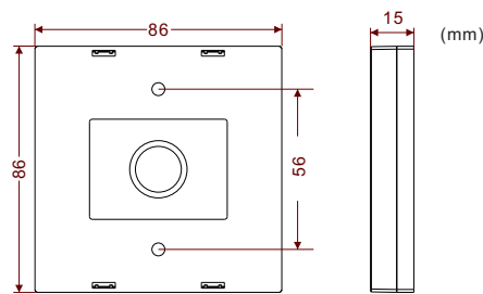
CNB-505M(明装款)
